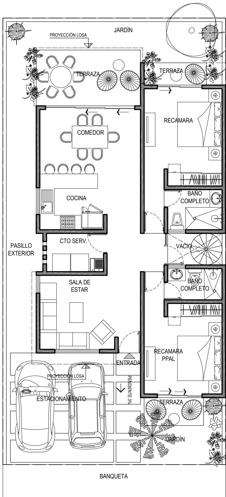
ARROLLO VEHICULAR PLANTA BAJA CASA CAMPO B ① ESCALA: 1:75
