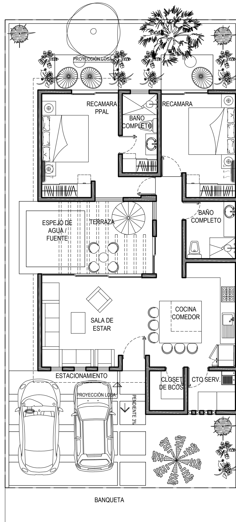
PLANTA BAJA CASA CAMPO ① ESCALA: 1:75
